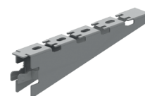
WKCL Console encliquetable à utiliser avec HSLE3 et profils perforés (trous oblongs 14x28mm)
